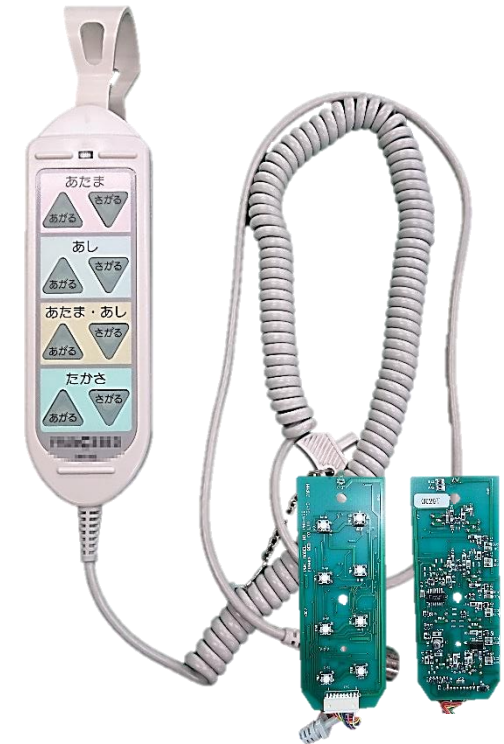
介護ベッド用リモコン
